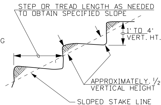
MINI BENCH DETAIL (SEE NOTE NOS. 2 & 6)
