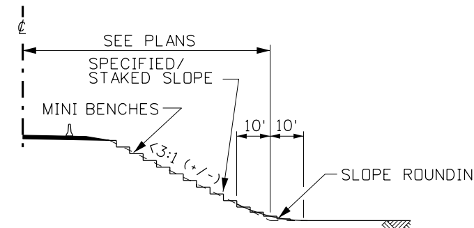
FILL SLOPES - 3:1 OR FLATTER
